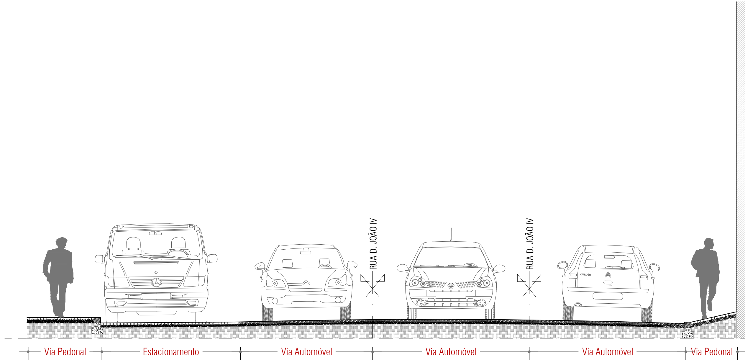
Perfil 2 Esc. 1:50
