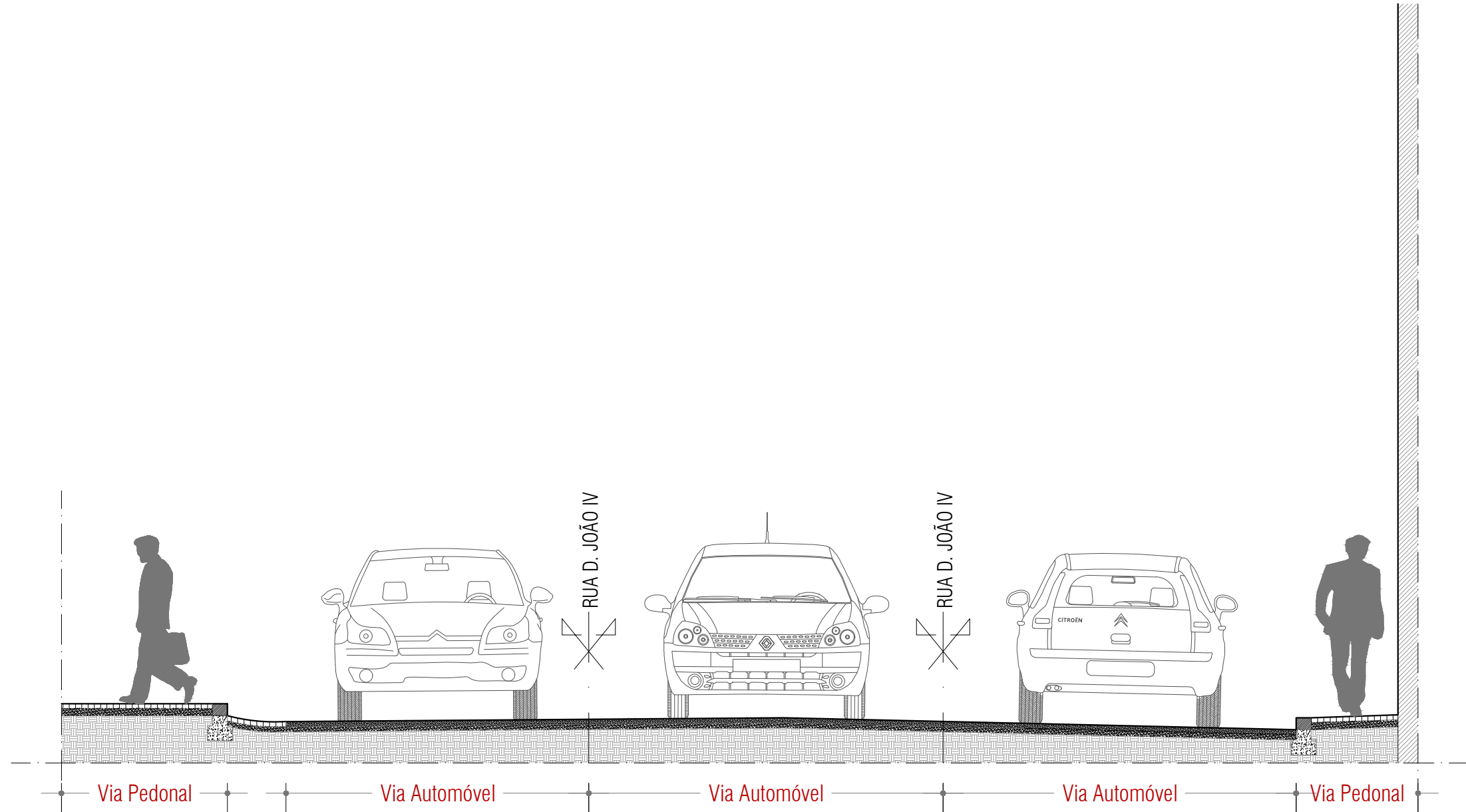
Perfil 1 Esc. 1:50
