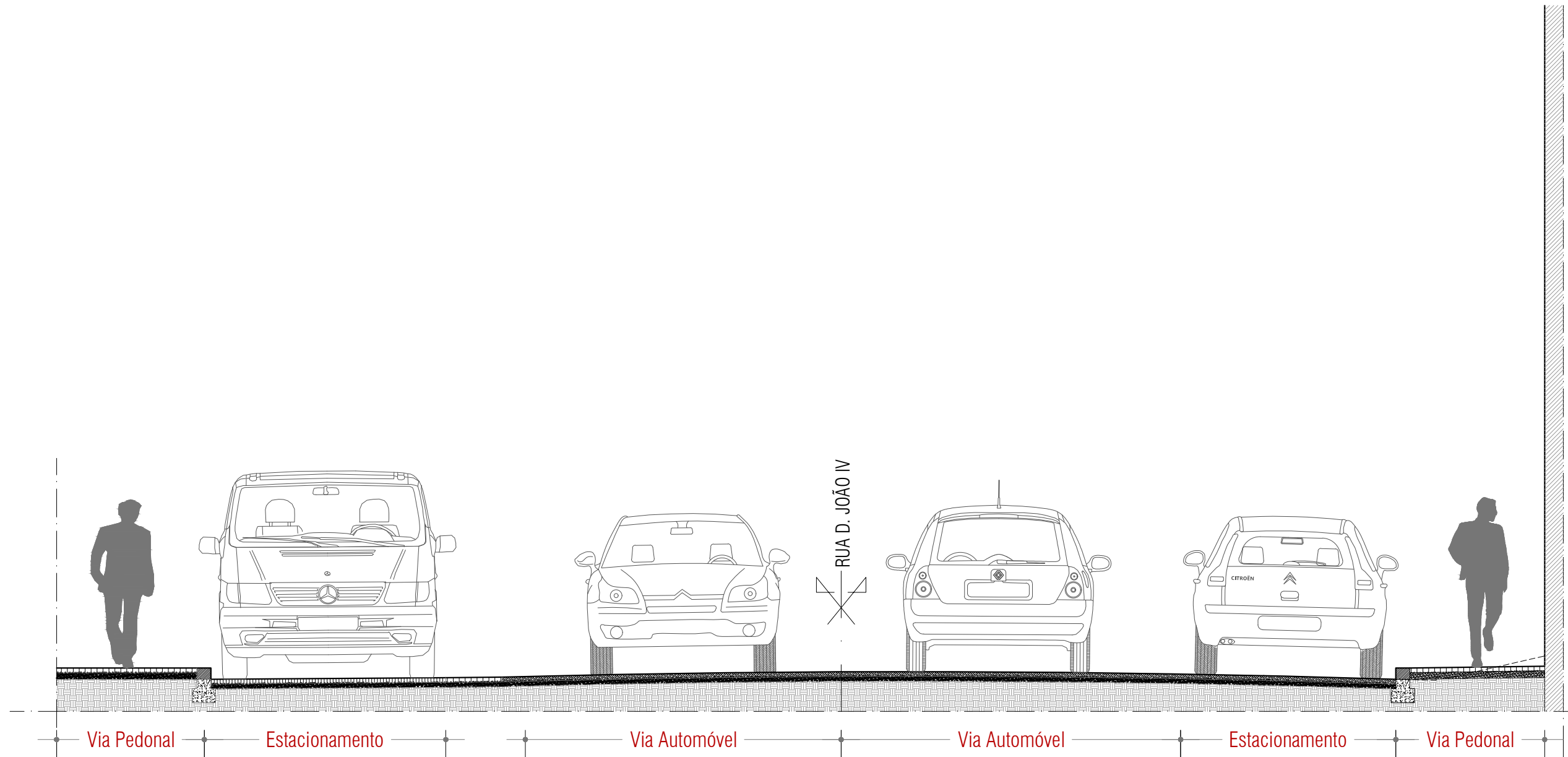
Perfil 2 Esc. 1:50
