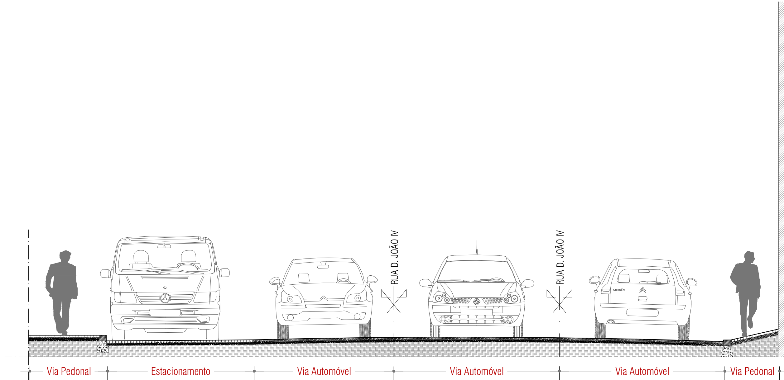
Perfil 2 Esc. 1:50
