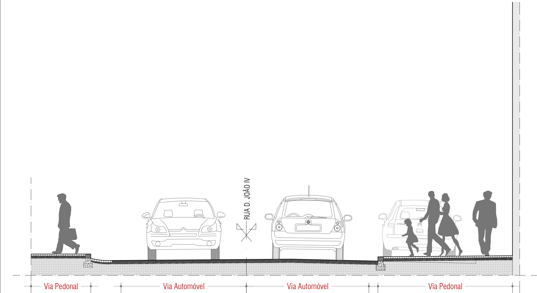
Perfil 1 Esc. 1:50
